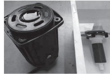
2. Pumpengehäuse 45° drehen im Gegenuhrzeigersinn (links) (nur DM30000S)
