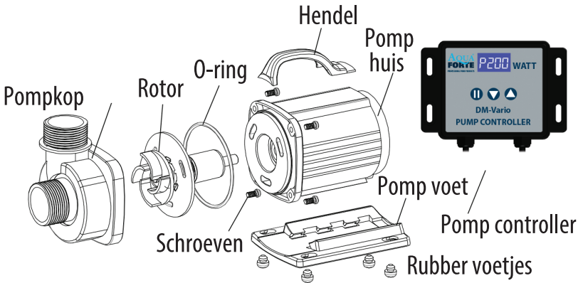
5. Zet pomphuis rechtop en vul deze met een milde ontkalker (zoals schoonmaakazijn). Leg de rotor in een plastic kom/bakje gevuld met hetzelfde anti-kalk middel en laat beiden 24 uur staan. Na 24 uur afspoelen met water en pomp weer assembleren.
